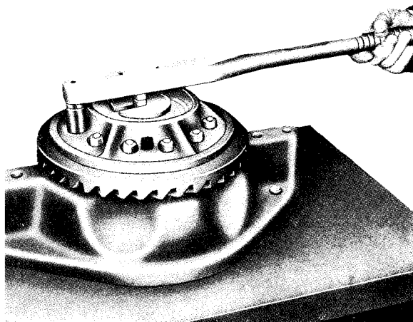
Sl. 9A.13 — Postavljanje tanjirastog zupčanika
