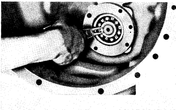
Sl. 8B.2 — Skidanje uskočnika i nosača ležaja
