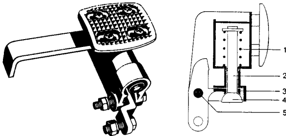
Sl. 11B.6 — Kompenzator aktiviranja
