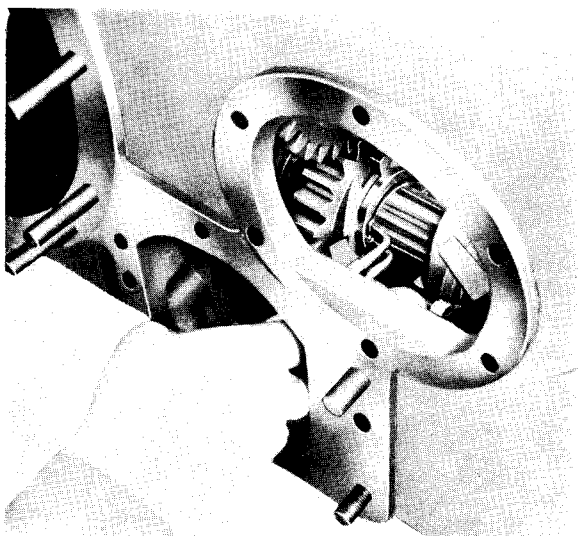
Sl. 10B.2 — Skidanje uskočnika
