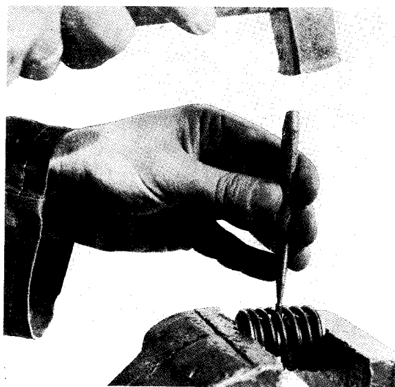
Sl. 13A.51 — Izbijanje elastične čivije
