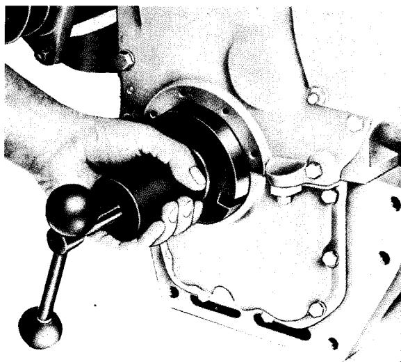
Sl. 2B.33 — Centriranje kućice zaptivače
