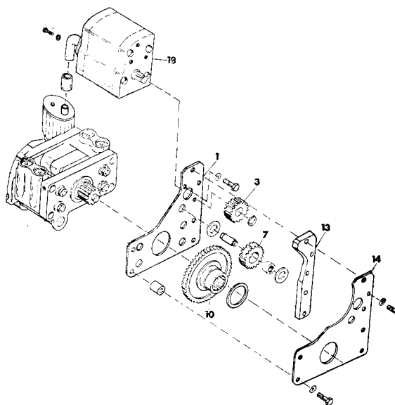
Sl. 13A.46 — Pumpa pomoćne hidraulike
