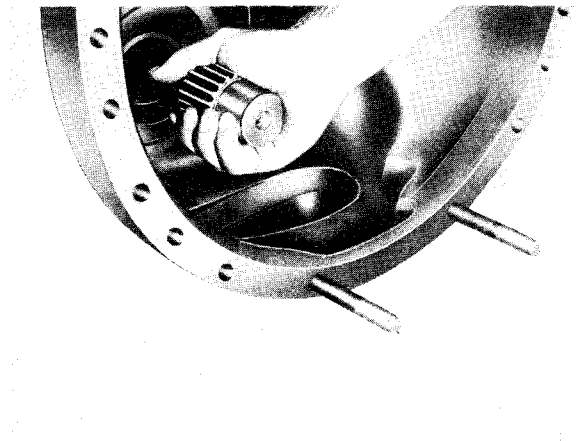
Sl. 8B.4 — Vađenje punog priključnog vratila
