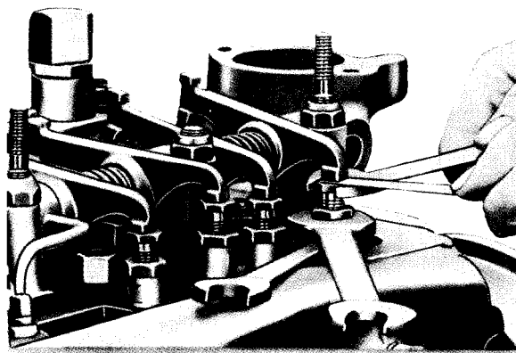
Sl. 2B.13 — Podešavanje zazora ventila
