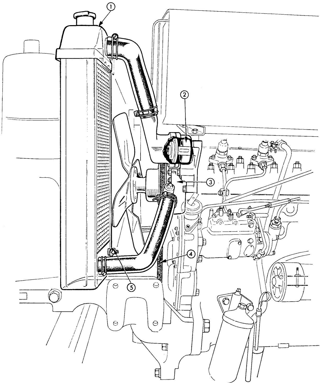
SI. 3A.1 — Opšti izgled sistema za hlađenje
