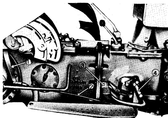
Sl. 11A.7 — Komande kočnica
