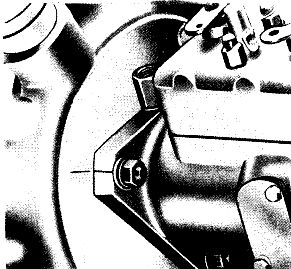
Sl. 2B.30 — Poravnavanje oznaka na kućištu razvoda i pumpi za ubrizgavanje
