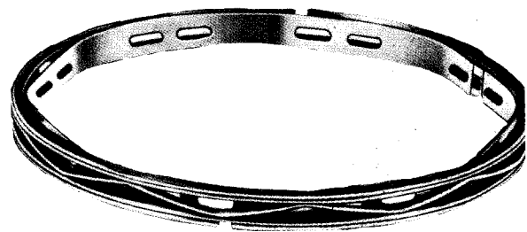
Sl. 2B.42 — Lamelasti klipni prsten-prvi uljni strugač
