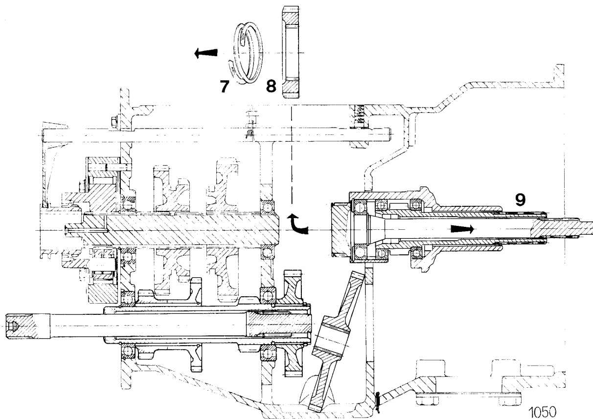
SI. 8C.6 — Skidanje sklopa punog i šupljeg ulaznog vratila
