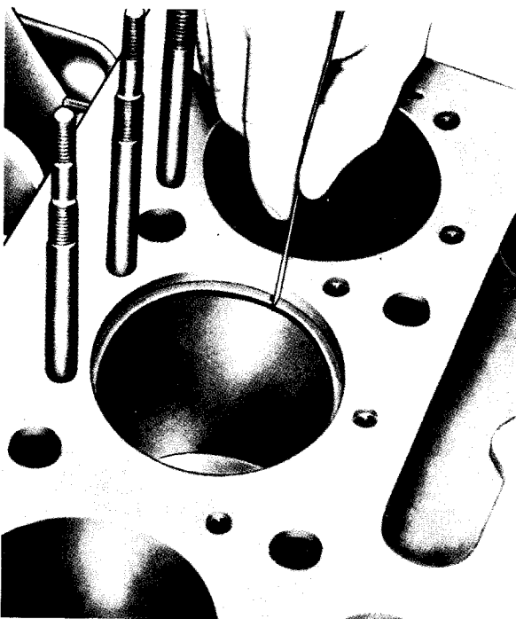
Sl. 2B.43 — Provera procepa krajeva klipnih prstenova
