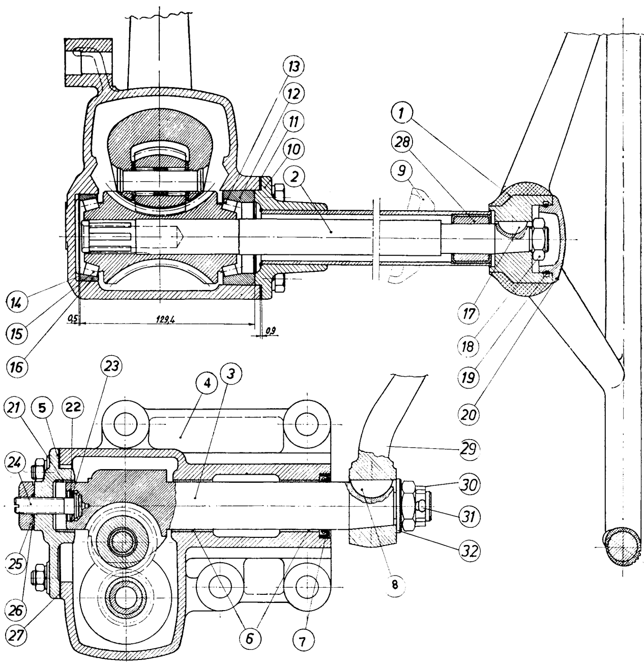
SI. 12A.1 — Uzdužni presek upravljača
