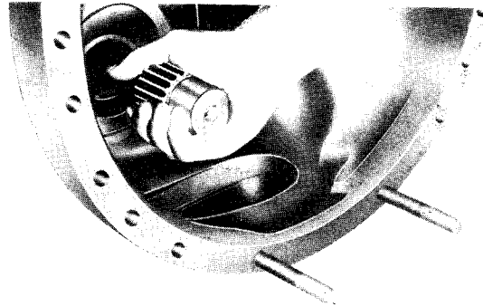
Sl. 8A.10 — Vadenje punog posrednog vratila
