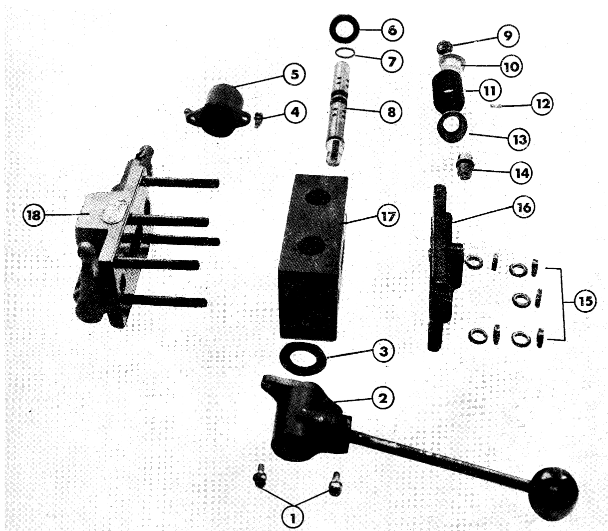
Sl. 13A.48 — Razvodnik pomoćne hidraulike
