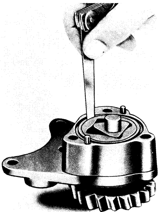
Sl. 2B.18 — Provera zazora između spoljnjeg rotora i tela pumpe za ulje
