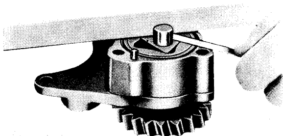
Sl. 2B.19 — Provera čeonog zazora pumpe za ulje
