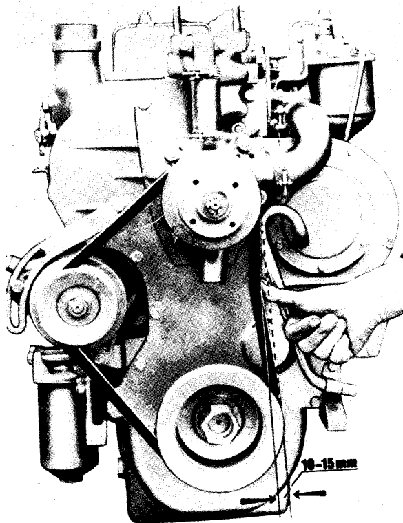
Sl. 3A.3 — Provera zategnutosti kaiša
