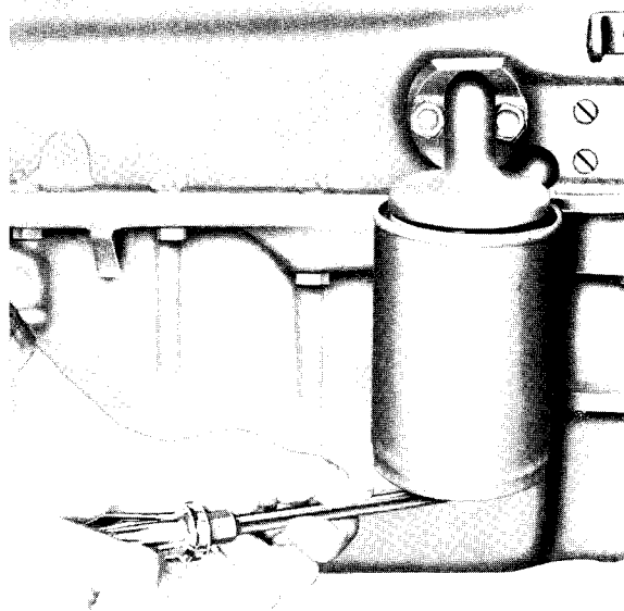
Sl. 2B.20 — Skidanje prečistača ulja
