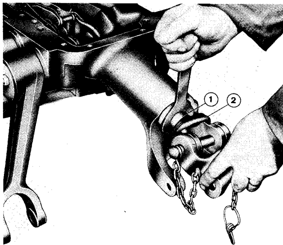
Sl. 13A.28 — Skidanje oslone navrtke balansne opruge
