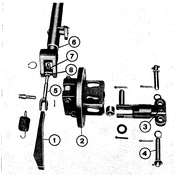
Sl. 11A.19 — Međusobni položaj delova mehanizma
