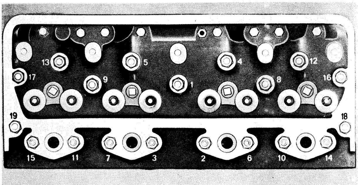
Sl. 2B.3 — Redosled pritezanja navrtki i zavrtnki glave cilindara
