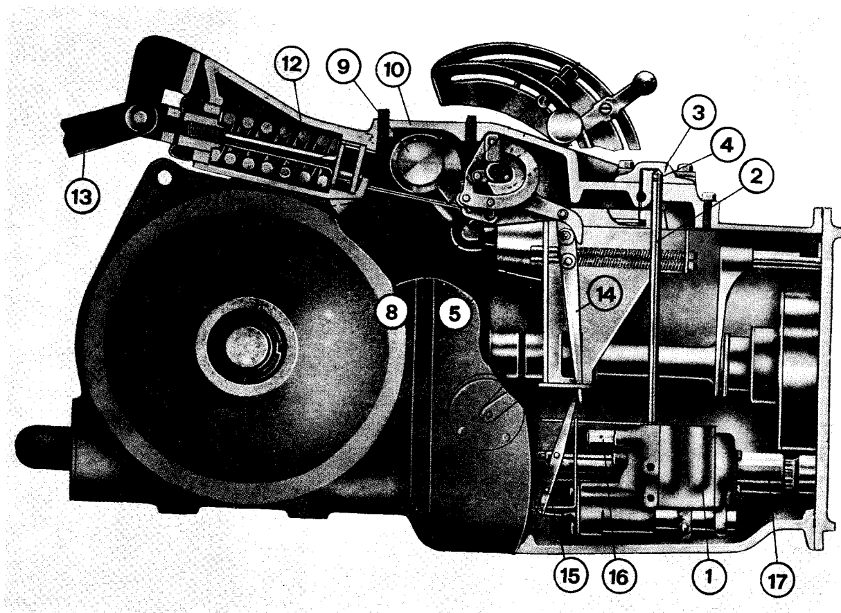
Sl. 13A.1 — Hidraulični podizni sistem (unutrašnji izgled)
