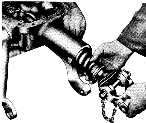
Sl. 13A.29 — Vadenje sklopa balansne opruge
