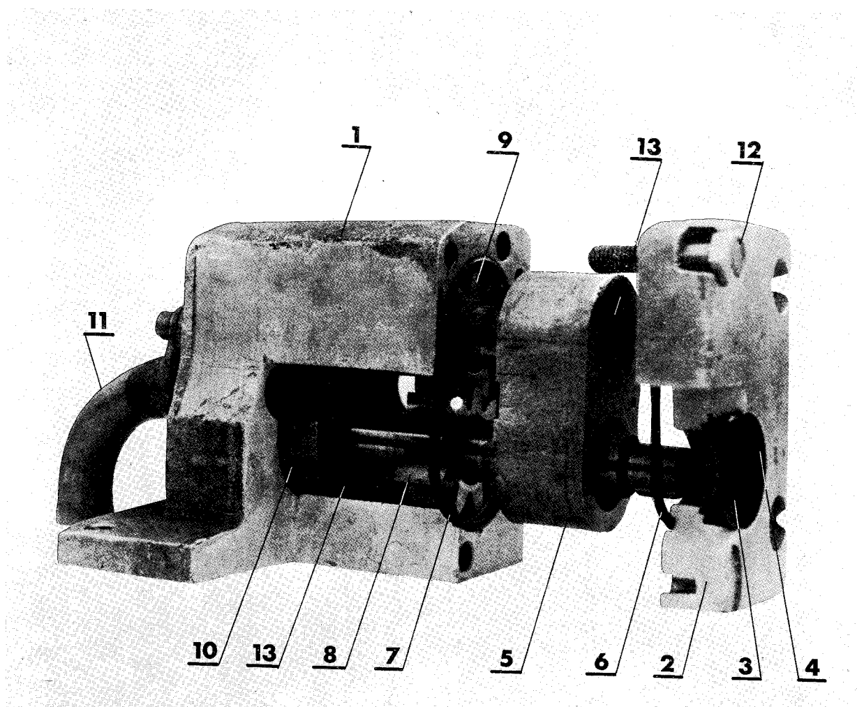
Sl. 13A.47 — Pumpa u rasklopljenom stanju
