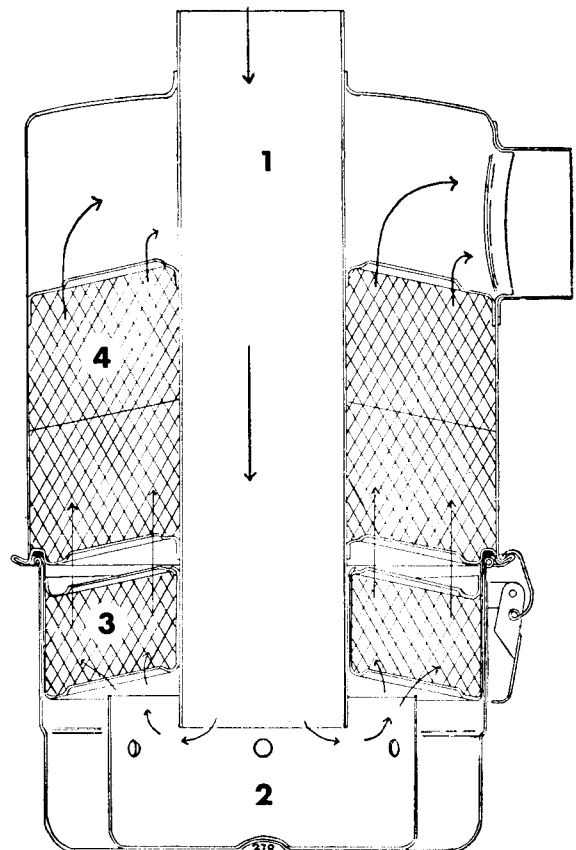
Sl. 4A.3 — Uzdužni presek kroz prečišćivač vazduha
