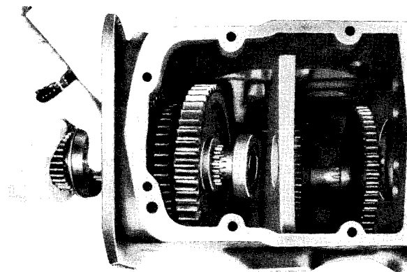
SI. 8A.17 — Vađenje glavnog vratila
