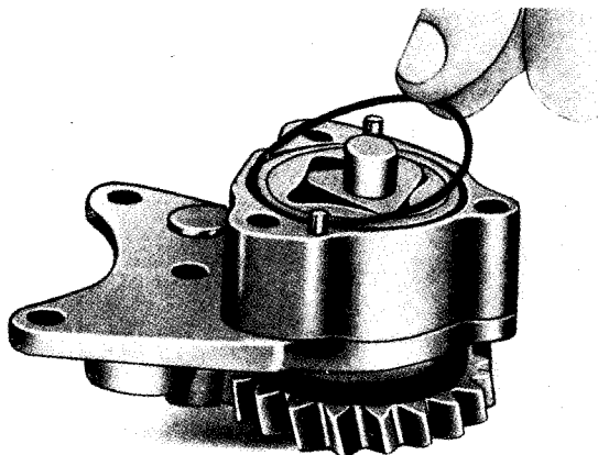
Sl. 2B.16 — Skidanje zaptivnog »C« prstena pumpe za ulje
