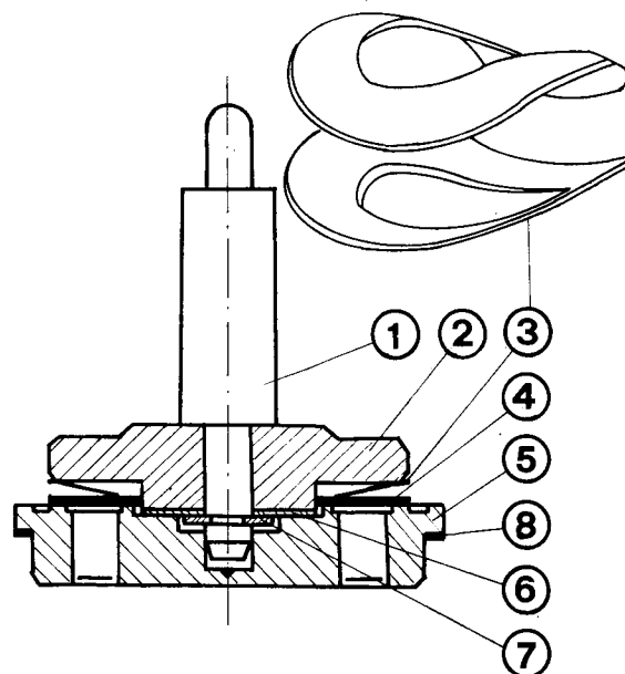
Sl. 11B.10 — Izgled preseka sklopa potisnog ventila refolement
