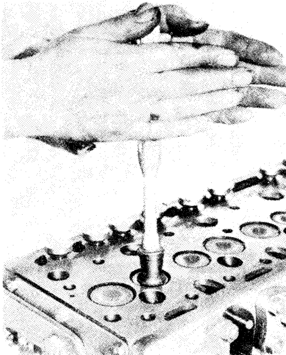
Sl. 2B.11 — Ručno brušenje ventila
