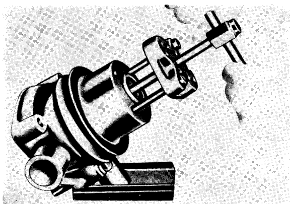
Sl. 3A.5 — Skidanje kaišnika pumpe za vodu
