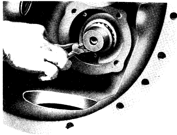
Sl. 8A.9 — Skidanje uskočnika
