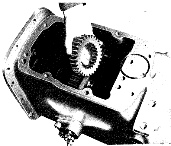
Sl. 8C.4 — Vadenje zupčanika
