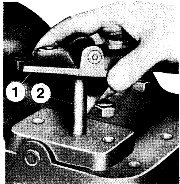
Sl. 13A.32 — Vadenje cevi uljnog voda
