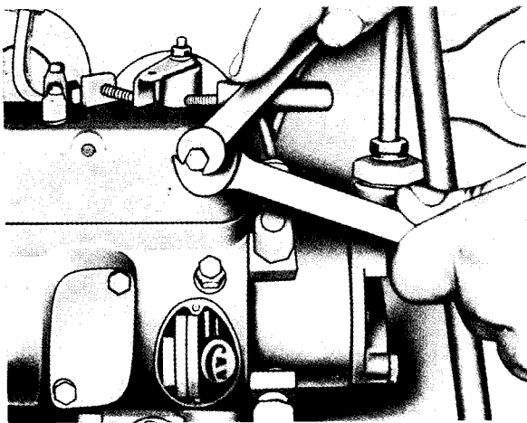
Sl. 2B.56 — Zavrtna na poklopcu regulatora pumpe
