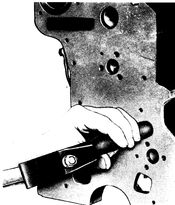
SI. 2B.47 — Utiskivanje slepog oka u blok
