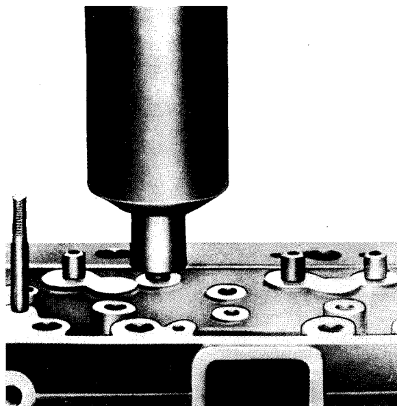
Sl. 2B.12 — Alat za utiskivanje vodica ventila
