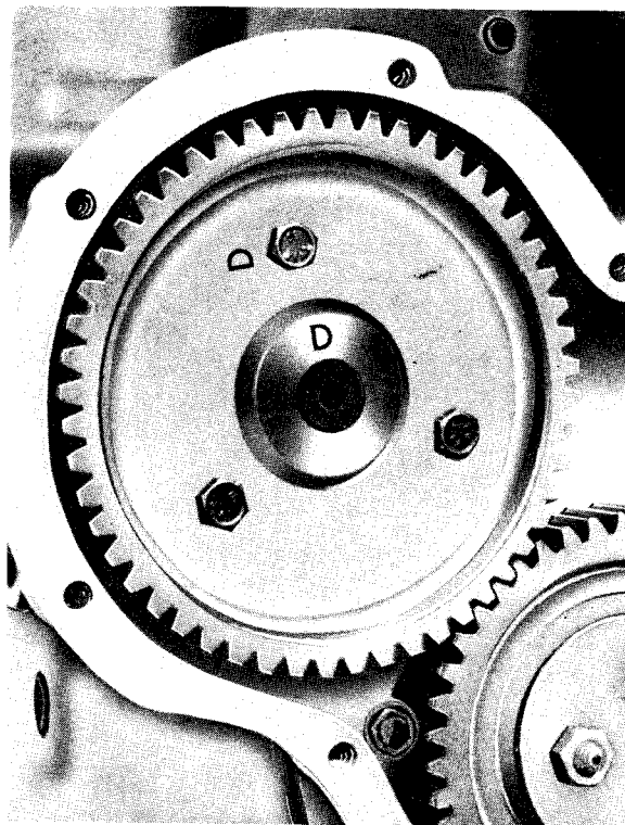
Sl. 2B.28 — Poravnavanje oznaka na vratilu i zupčanicu
