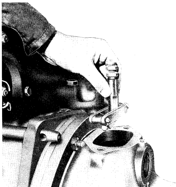
Sl. 11A.2 — Vađenje mehanizma kočnice
