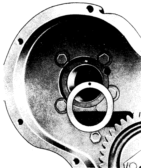
Sl. 2B.27 — Oslona ploča bregastog vratila
