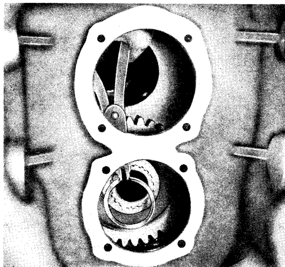
Sl. 8A.19 — Skidanje uskočnika sa šupljev posrednog vratila
