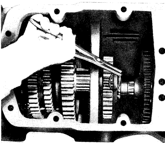
SI. 8A.16 — Skidanje uskočnika sa glavnog vratila
