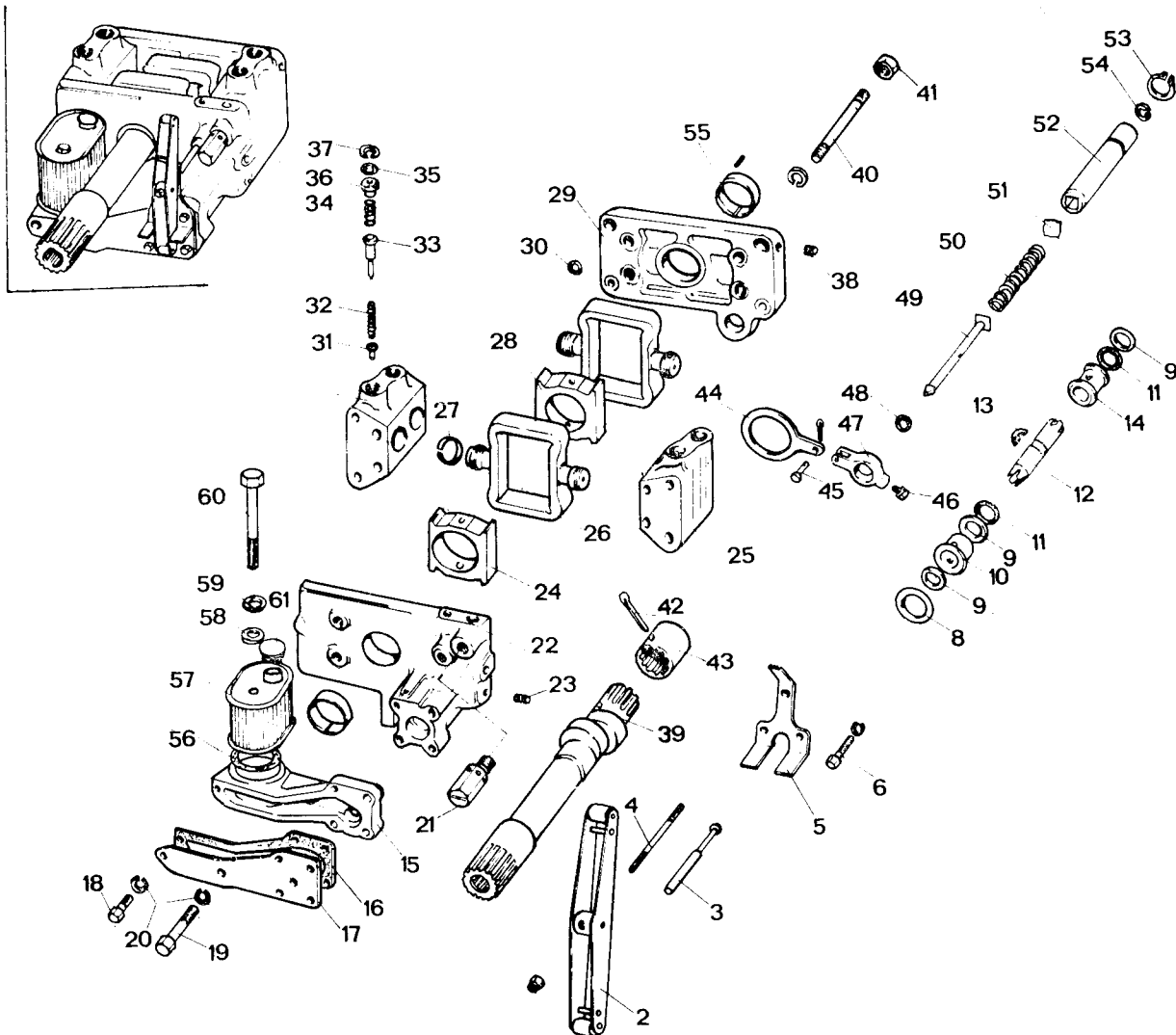
Sl. 13A.41 — Izgled rastavljenog sklopa hidraulične pumpe
