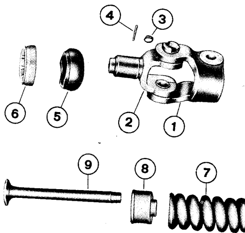
Sl. 13A.30 — Izgled rasklopljenog sklopa balansne opruge
