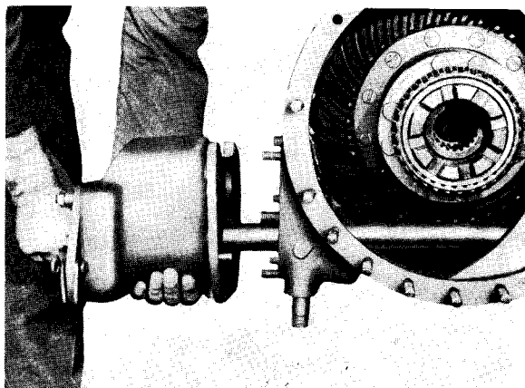
Sl. 10B.3 — Skidanje zadnjeg priključnog vratila
