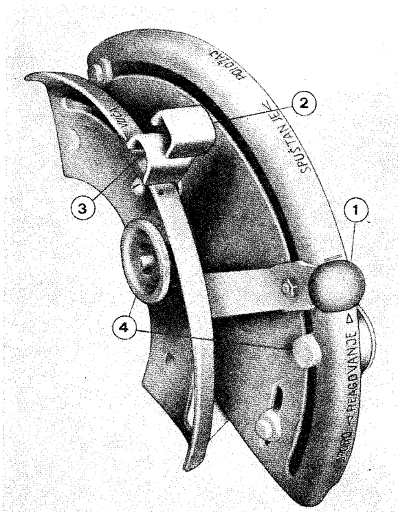
Sl. 13A.21 — Komandne ručice na sektorskim oznakama
