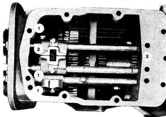
Sl. 8A.5 — Šipke menjača i reduktora
