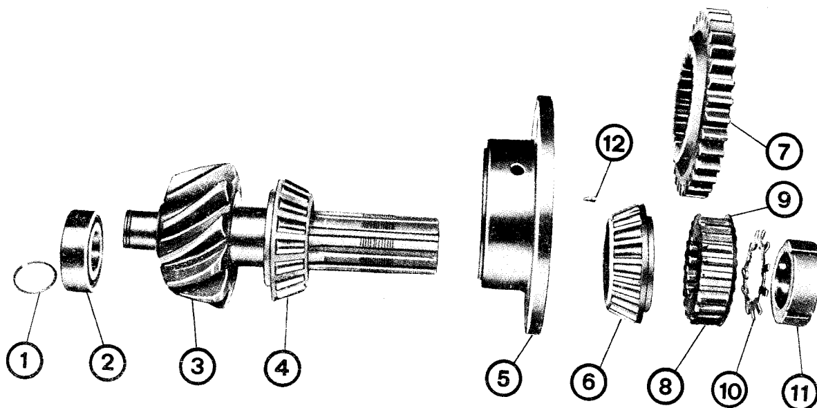
Sl. 9A.11 — Pogonski zupčanik i nosač — sklop
