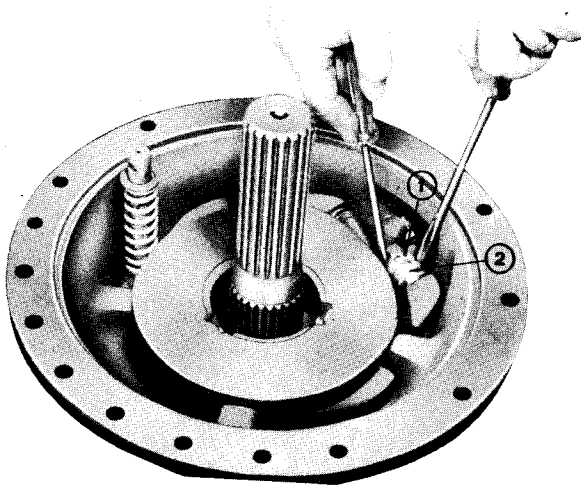
Sl. 11A.10 — Vađenje kočionog cilindra 1. Zavrтка 2. Navrtka za osiguranje
