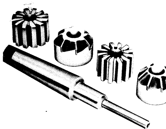
Sl. 2B.7 — Alat za obradu sedišta ventila
