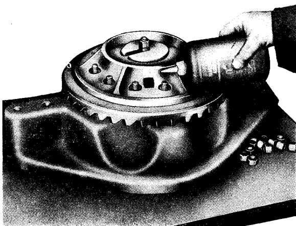
Sl. 9A.12 — Osiguranje navoja zavrtnjeva
