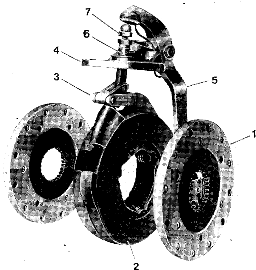
Sl. 11A.5 — Međusobni položaj komponenti sklopa
