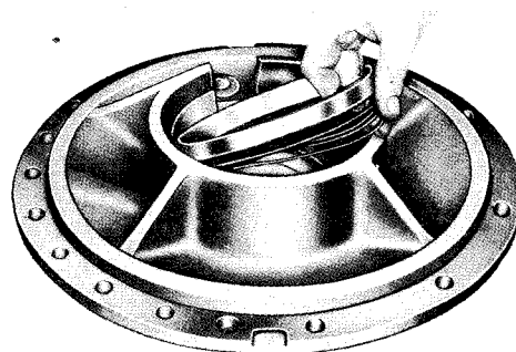
Sl. 9A.25 — Stavljanje podloški za podešavanje
