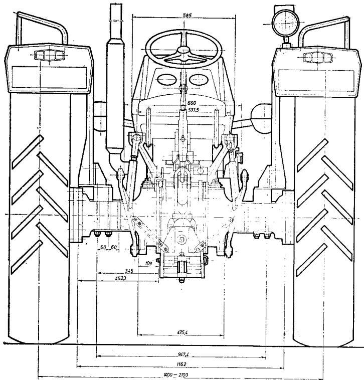
Sl. 1A.2 — Glavne mere traktora (IMT-560)
