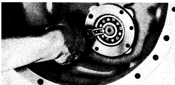
Sl. 8C.2 — Skidanje uskočnika
