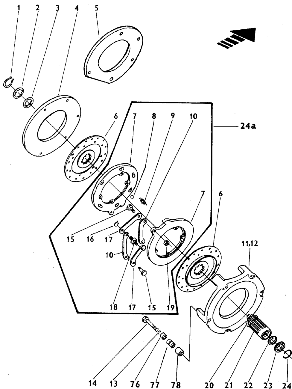
26a NOŽNÍ BRZDA DISKOVÁ - SCHEIBENFUSSBREMSE - DISK TYPE FOOT BRAKE - FREIN À PÉDALE À DISQUE - FRENO DE PEDAL DE DISCO (7245-2600/08) 26a
